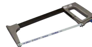
▲ Arco para serra de metal Irimo Profissional e robusto Montagem alternativa a 55° para corte biselado Inclui serra bi-metal 24 dpp Ref. 20436
